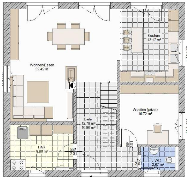
Erdgeschoss
